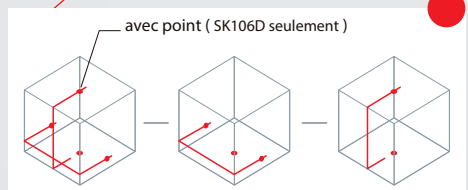
FAISCEAU ROUGE SK105D / SK106D
